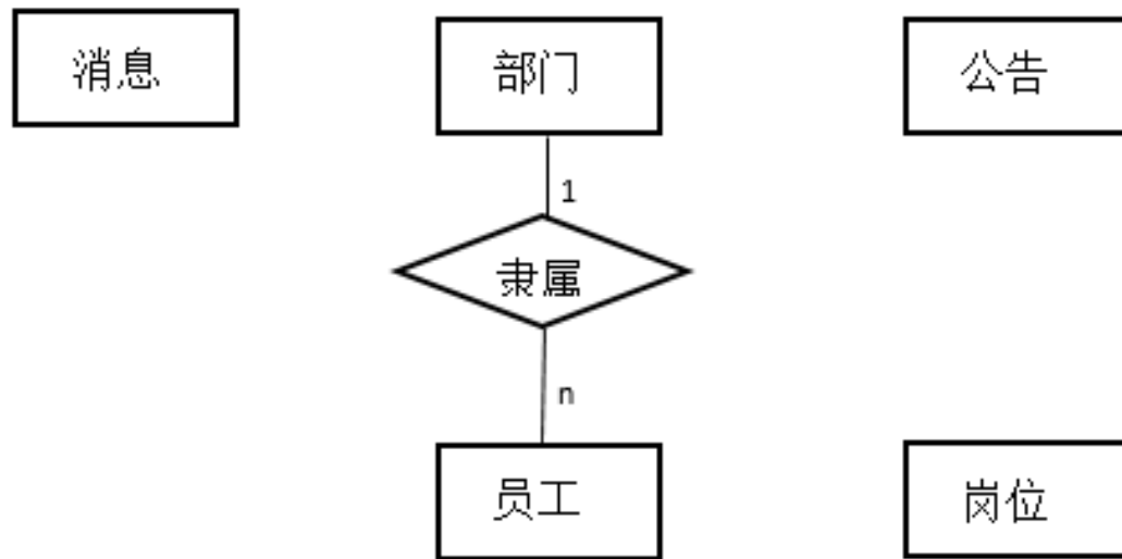
图 2-1 实体联系图
