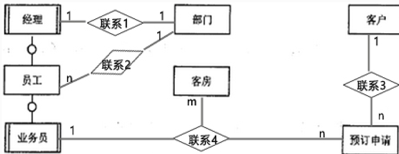
图 2-1 实体联系图
